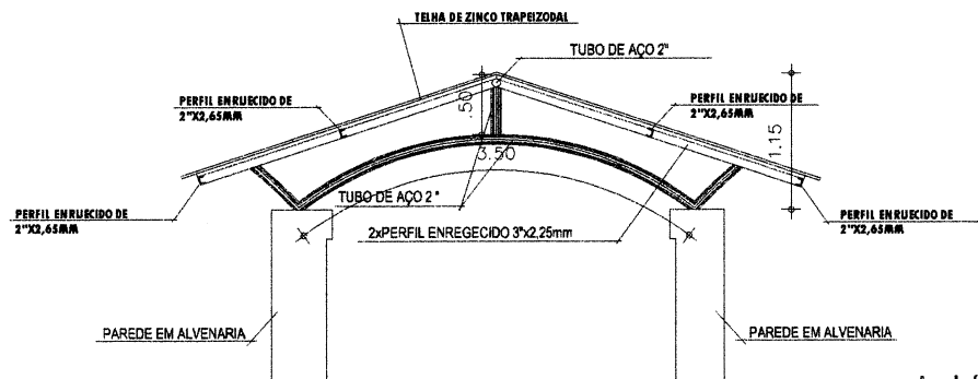
DETALHE COBERTA EM TELHA DE ZINCO ESC 1:50
