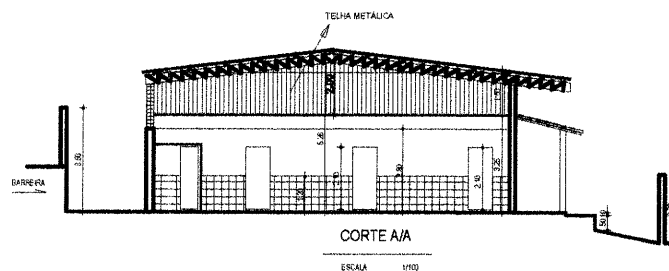
MODELO DA COBERTA
