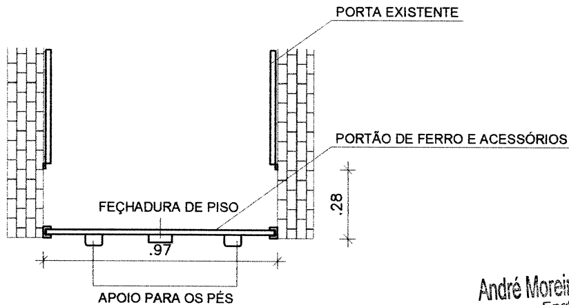
PLANTA BAIXA DO PORTÃO
