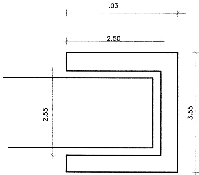
DETALHE DA CANTONEIRA
