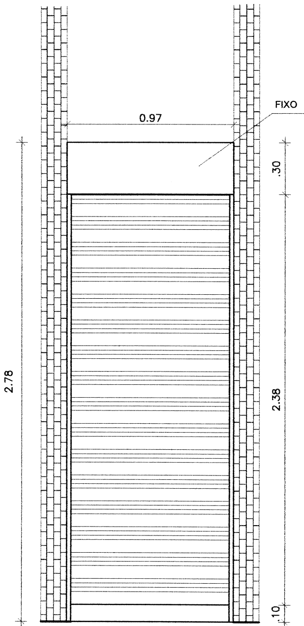
ELEVAÇÃO DO PORTÃO DE FERRO
